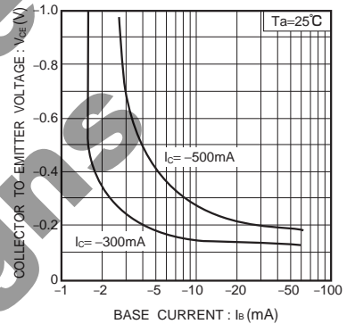
Fig.6 コレクタ・エミッタ間飽和電圧 —ベース電流特性
