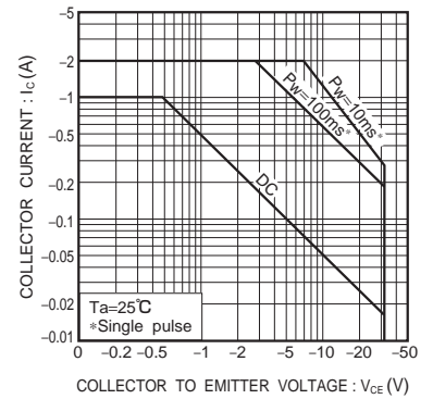
Fig.9 安全動作領域 (2SB1132)
