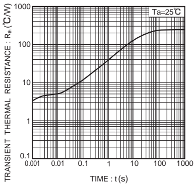
Fig.10 過度熱抵抗 (2SB1132)
