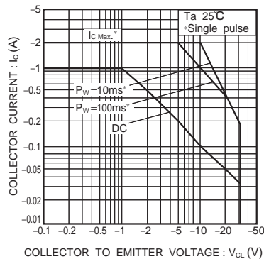
Fig.11 安全動作領域 (2SB1237)
